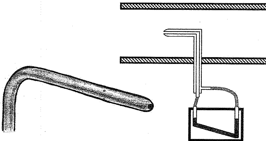
Figura N°8: Tubo de Pitot
