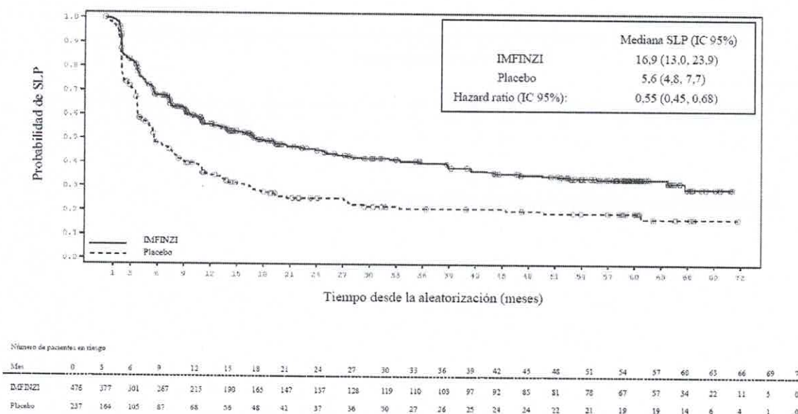
Figura 2. Curva de Kaplan-Meier de la PFS (DCO 11 Jan 2021)
