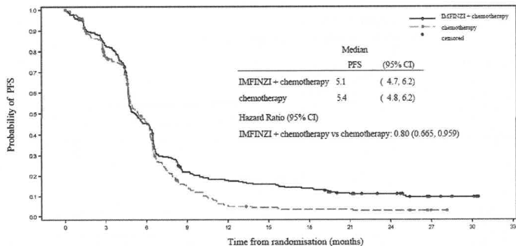
Figura 9. Curva Kaplan-Meier de PFS (DCO 27 Ene 2020)
