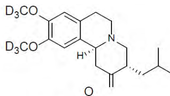
SS - Deutetrabenazina
